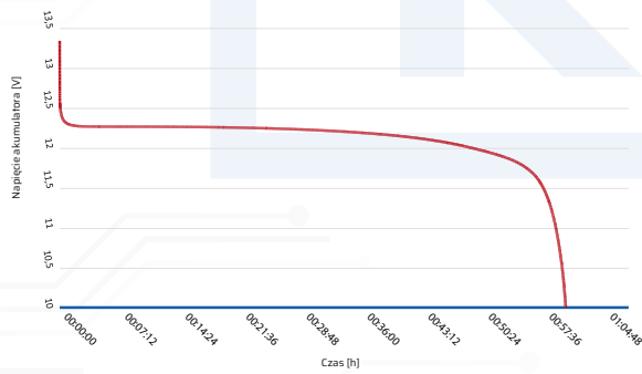
Rys. 1 Spadek napięcia na akumulatorze, rozładowanie 1C
