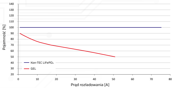
Rys. 5. Porównanie pojemności akumulatorów Kon-TEC LiFePO4 i kwasowo-olowiowych, przy różnych prądach rozładowania
